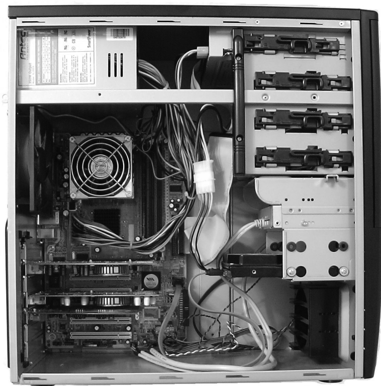
Figura 4.1: Gabinete aberto
